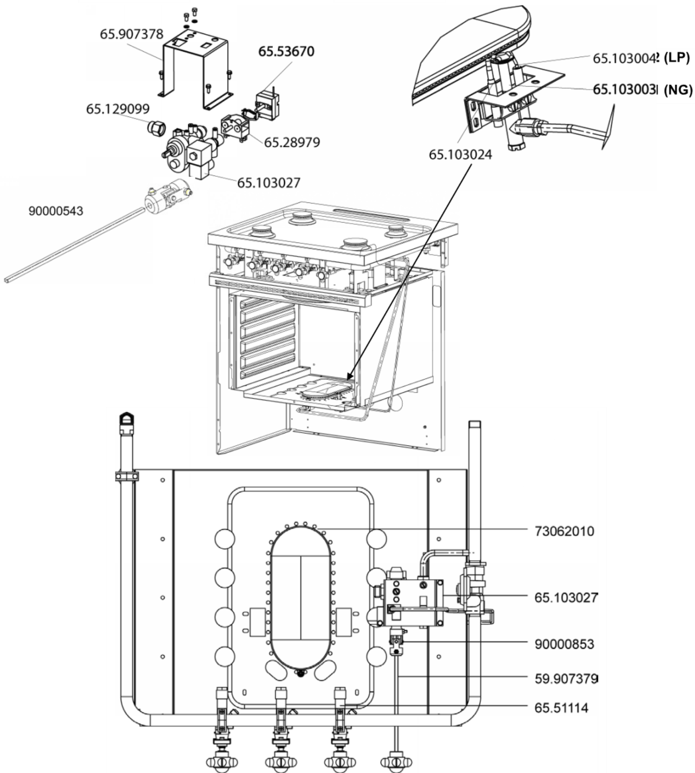
Détail A:
