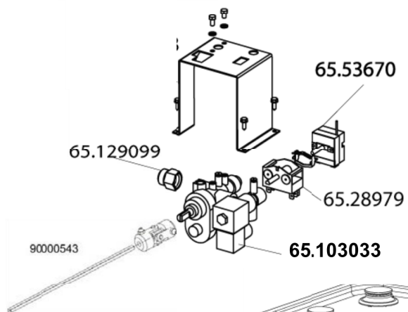
Détail A :
